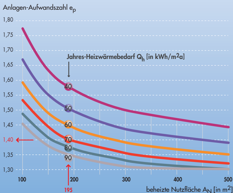
Bild 5: Mit dem Diagrammverfahren nach DIN V 4701-10 lässt sich die Anlagen-Aufwandszahl einfach ermitteln.
