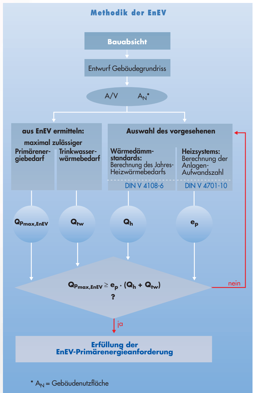
Bild 4: Methodik der EnEV
